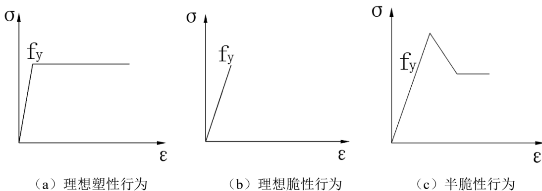
图 3.3 理想状态下钢材单向拉伸应力—应变曲线
