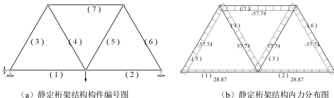
图 5.1 静定钢桁架结构图
