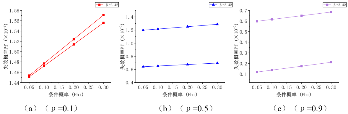
图 5.6 结构失效概率与条件概率关系曲线 ( n=47 )
