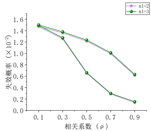
(b) 不同潜在脆性破坏构件个数
