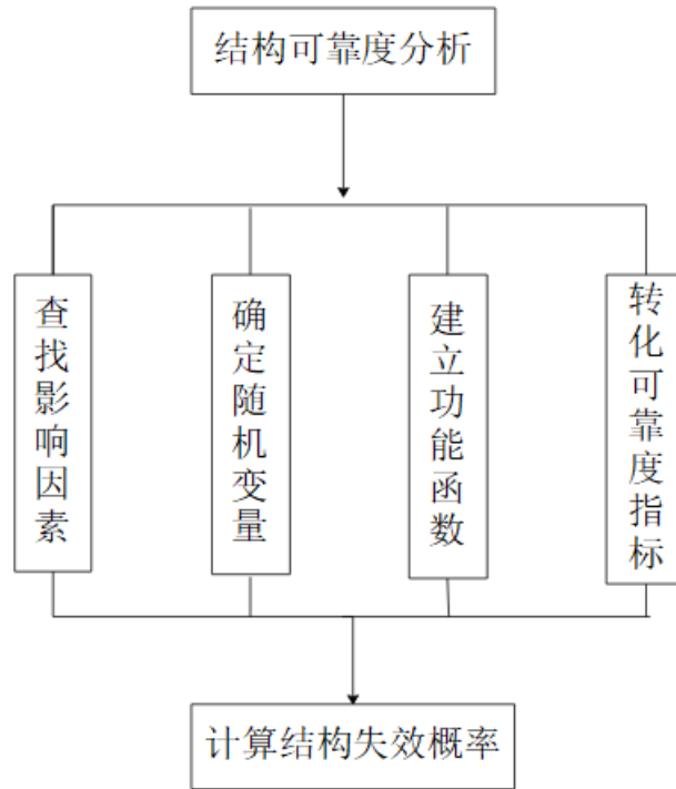
图 2.2 结构可靠性分析流程示意图
