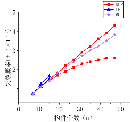
(b) 构件个数与失效概率关系曲线图 ( \rho=0.5 )
