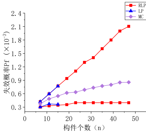
(c) 构件个数与失效概率关系曲线图 ( \rho=0.9 )
