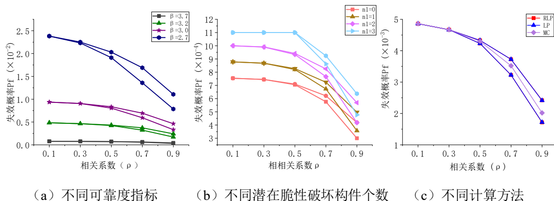
图 4.9 结构失效概率与相关系数关系曲线
