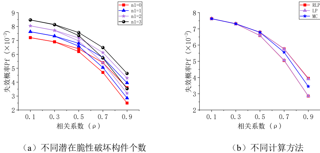
图 5.3 结构失效概率与相关系数关系曲线 ( n=7 )
