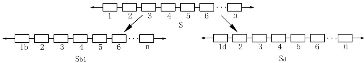
图 3.6 构件 1 为潜在脆性破坏构件的结构系统分析示意图
