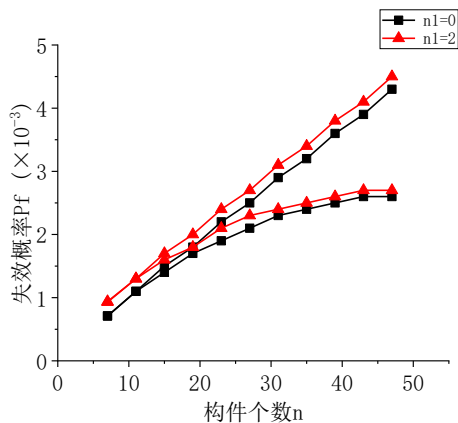
(c) 构件总数与失效概率关系曲线图
