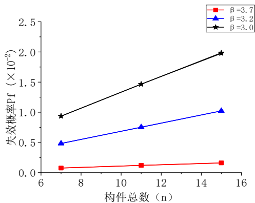
(a) 构件总数与结构失效概率关系曲线 ( \rho=0.1 )
