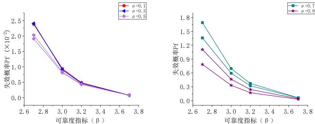
图 4.7 结构失效概率与可靠度指标关系曲线（不同相关系数）
