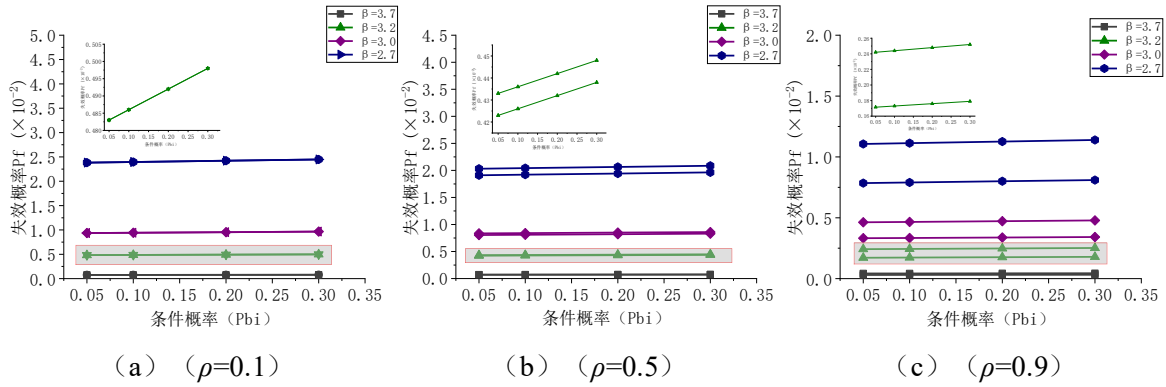
图 4.1 不同可靠度指标条件下结构失效概率与条件概率关系曲线
