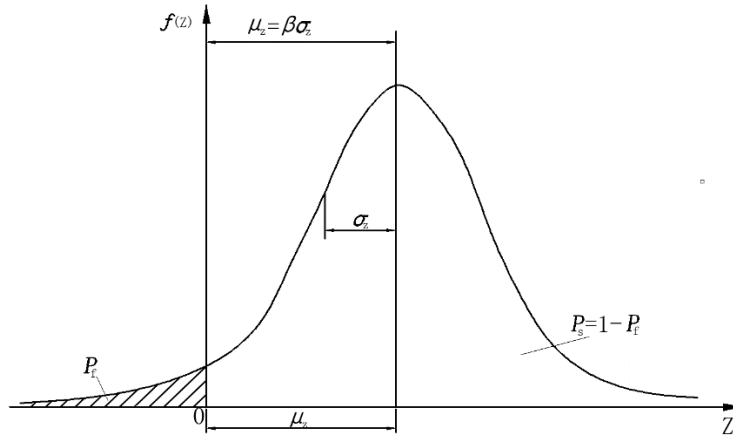
图 2.3 失效概率与可靠度指标的关系
