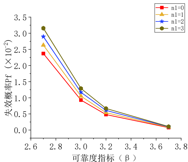
图 4.8 结构失效概率与可靠度指标关系曲线（不同潜在脆性破坏构件个数）
