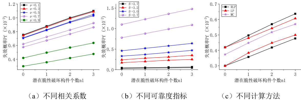
图 4.10 结构失效概率与潜在脆性破坏构件个数关系曲线
