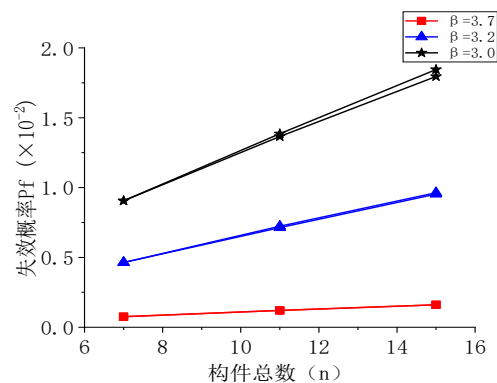
(b) 构件总数与结构失效概率关系曲线 ( \rho=0.3 )
