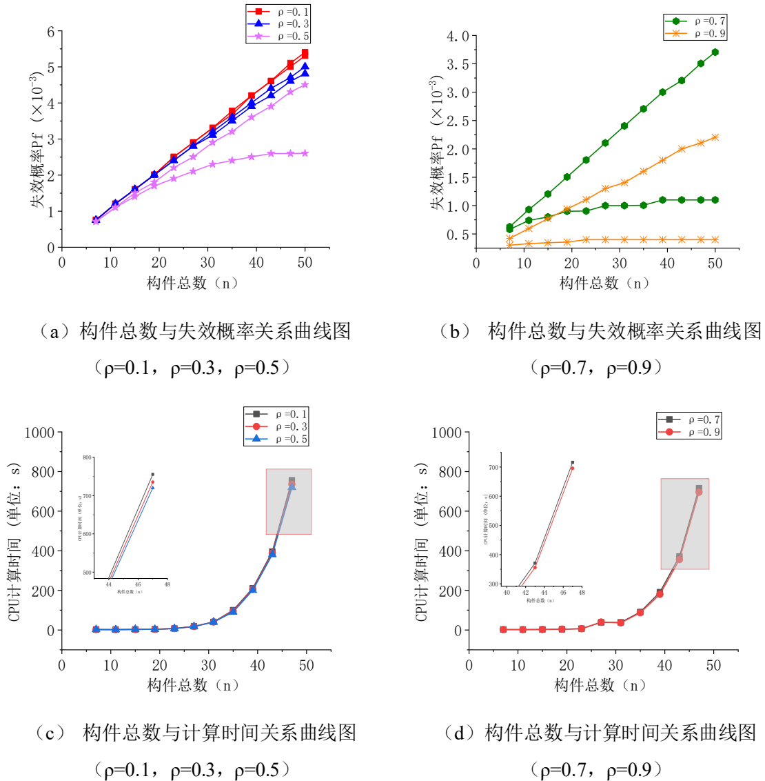
图 4.5 构件总数与结构失效概率关系及计算效率曲线 (不同相关系数)
