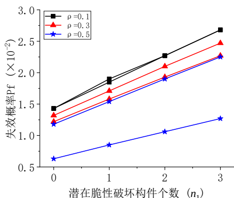
(a) 不同相关系数 ( \rho=0.1 \rho=0.3 \rho=0.5 )
