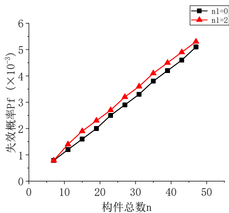
(a) 构件总数与失效概率关系曲线图
