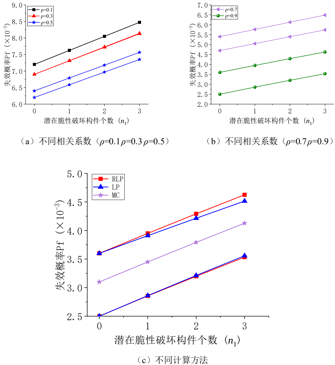
图 5.4 结构失效概率与潜在脆性破坏构件个数系曲线 ( n=7 )
