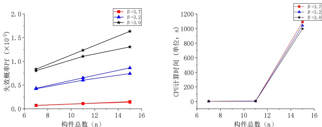
(c) 构件总数与结构失效概率关系曲线图 ( \rho=0.5 ) (d) 构件总数与计算时间的关系曲线图
