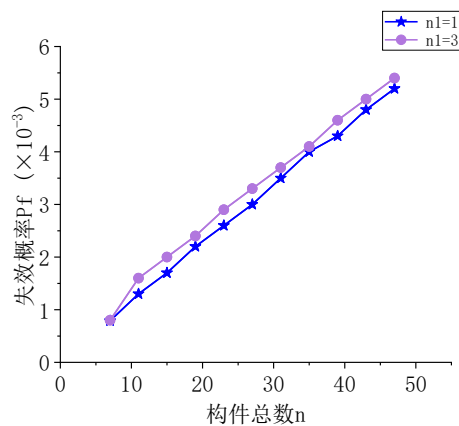
(b) 构件总数与失效概率关系曲线图
