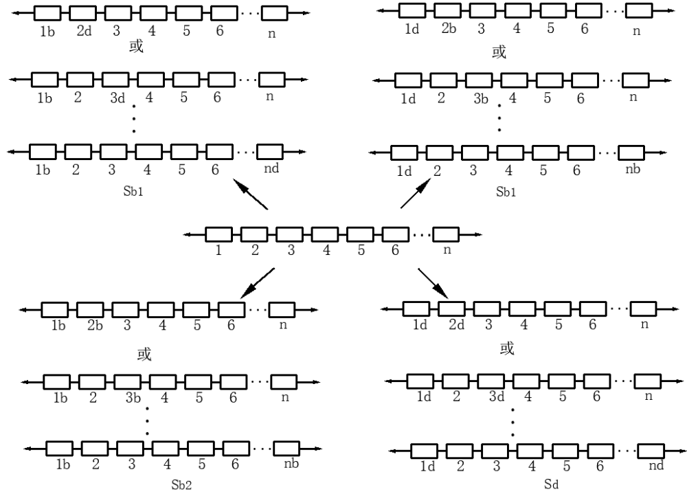
图 3.9 含两个潜在脆性破坏构件的结构系统分析示意图
