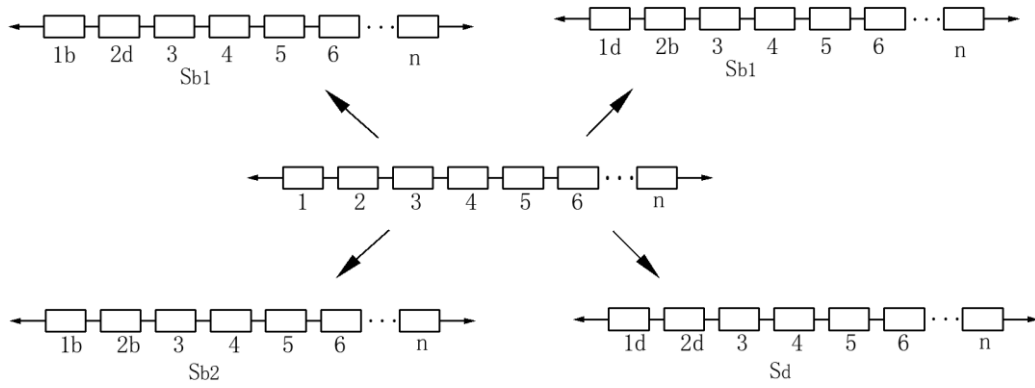
图 3.8 构件 1、2 为潜在脆性破坏构件的结构系统分析示意图
