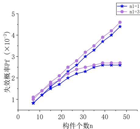
(d) 构件总数与失效概率关系曲线图
