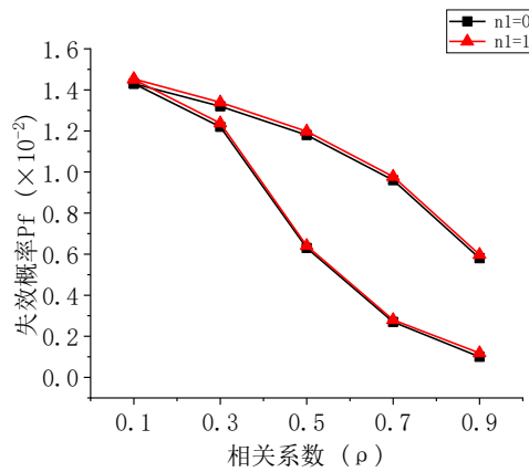
(a) 不同潜在脆性破坏构件个数
