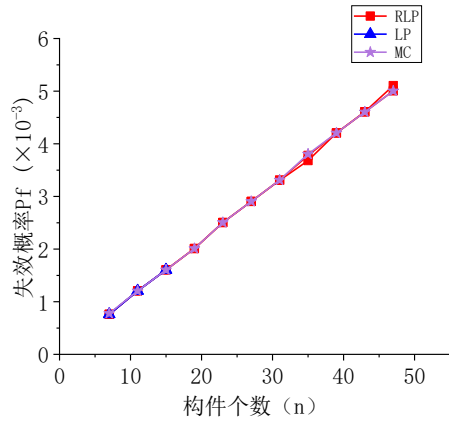
(a) 构件个数与失效概率关系曲线图 ( \rho=0.1 )
