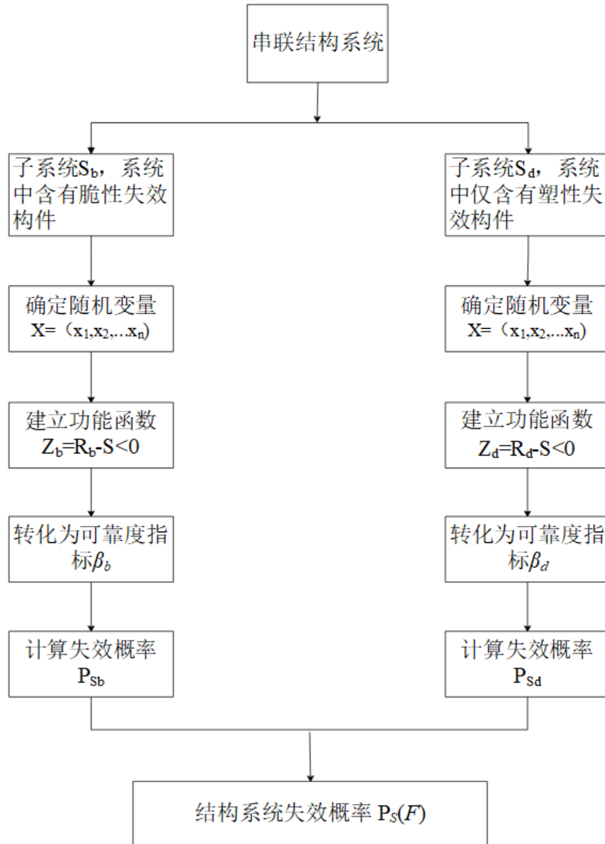
图 3.5 含潜在脆性破坏构件的结构体系失效概率计算流程图
