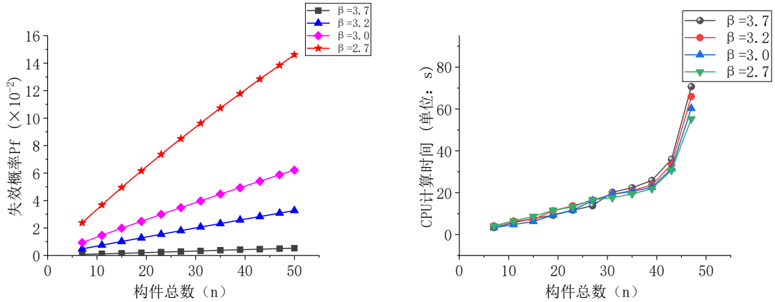
(a) 构件总数与失效概率关系曲线图 ( \rho=0.1 ) (b) 构件总数与计算时间的关系曲线图
