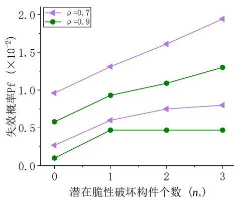
(b) 不同相关系数 ( \rho=0.7 \rho=0.9 )
