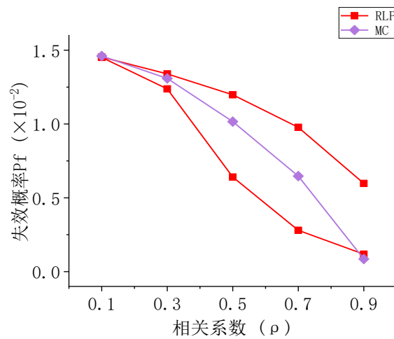
(c) 不同计算方法
