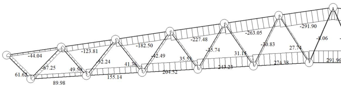
(b) 屋架结构内力图 (左半部分)
