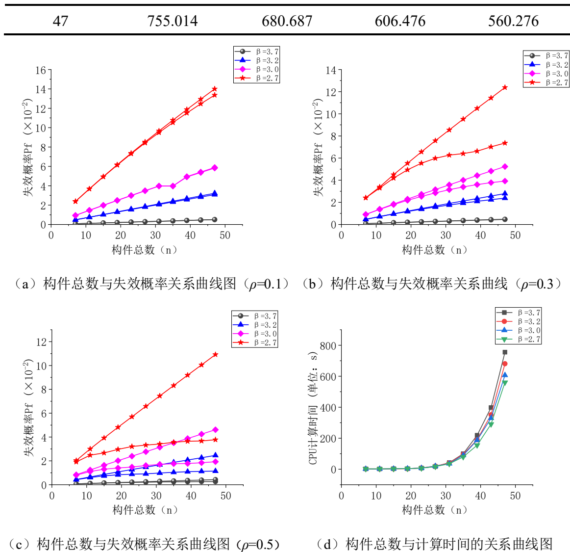
图 4.3 构件总数与结构失效概率关系及其效率 (RLP 方法)
