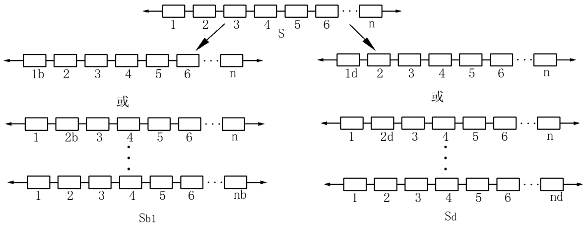
图 3.7 含一个潜在脆性破坏构件的结构系统分析示意图
