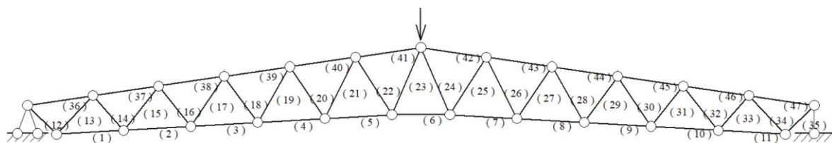
(a) 屋架结构构件编号图
