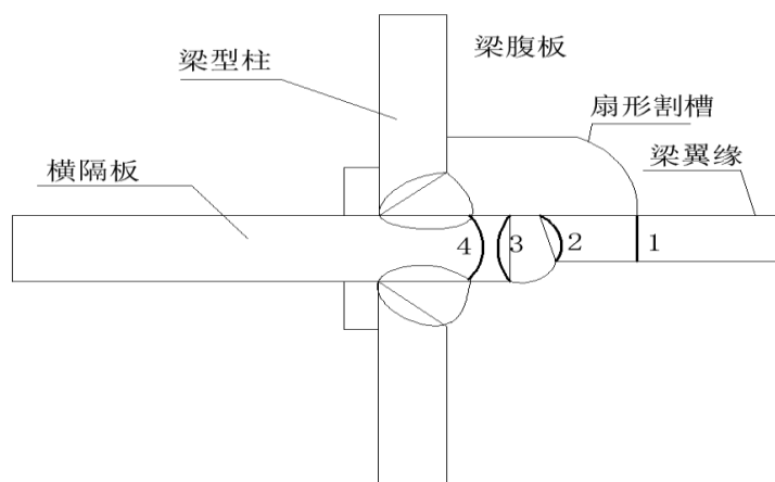
图 3.1 阪神地震梁柱节点破坏模式
